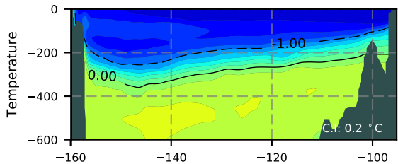
BCTGE28ERA5SC1 / Beaufort Section 1982
