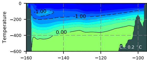
BCTGE28ERA5SC1 / Beaufort Section 2008
