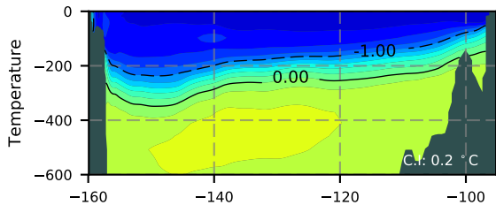
ERA01NEM405RGB / Beaufort Section 1989
