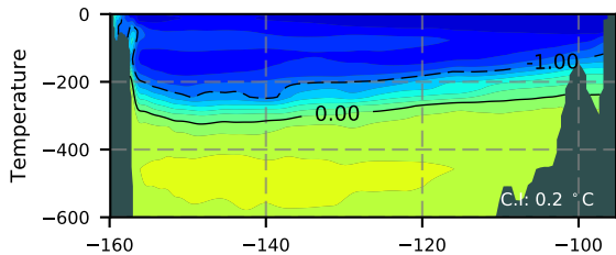
NEMO420 / Beaufort Section 1980
