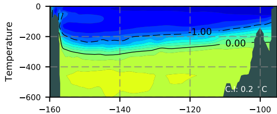
NEMO420 / Beaufort Section 1981
