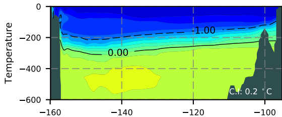
NEMO420 / Beaufort Section 1984
