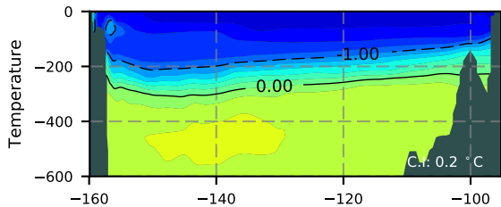
NEMO420 / Beaufort Section 1985
