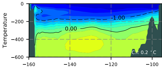
NEMO420 / Beaufort Section 1992
