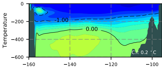
NEMO420 / Beaufort Section 2006
