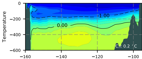
NEMO420IRW / Beaufort Section 1992
