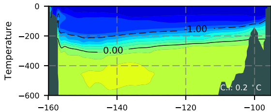
NEMO420WND / Beaufort Section 1984
