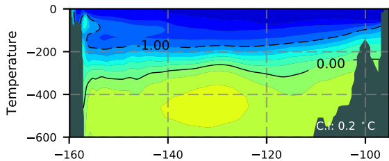
NEMO420WND / Beaufort Section 1992
