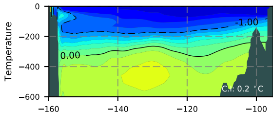
NEMO420WND / Beaufort Section 1993
