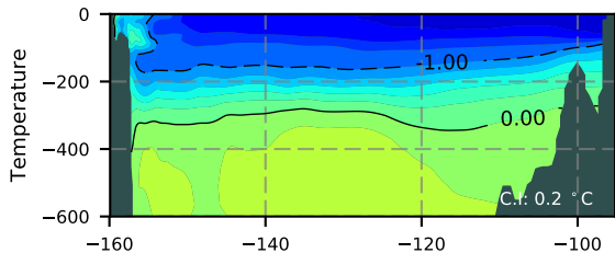
NEMO420WND / Beaufort Section 1998
