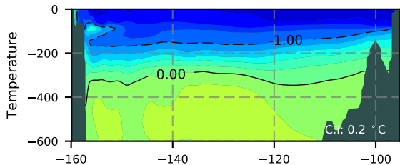
NEMO420WND / Beaufort Section 1999
