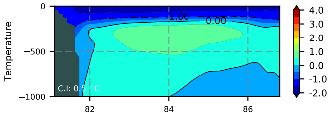
NEMO420WND / Kara Section 1987
