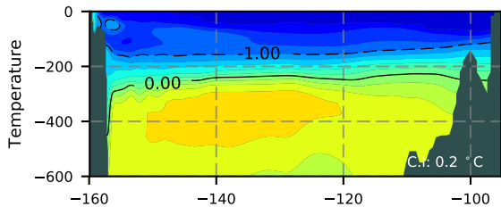
BCTGE28 / Beaufort Section 1990
