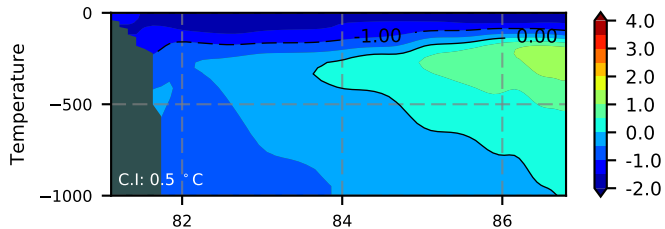
BCTGE28 / Kara Section 2011
