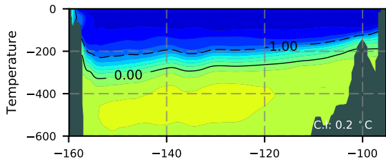
BCTGE28SSBDY / Beaufort Section 1990
