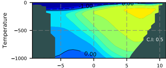
BCTGE28SSBDY / FramS Section 1996
