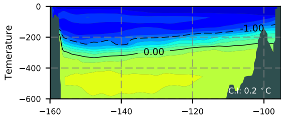
BCTGE26 / Beaufort Section 1960
