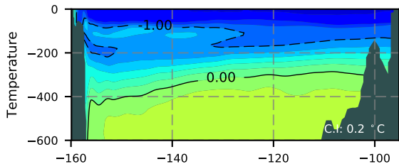
ILBOXE68 / Beaufort Section 2013
