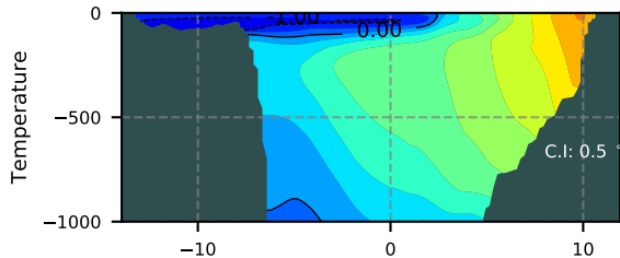
FUT08 / FramS Section 2070
